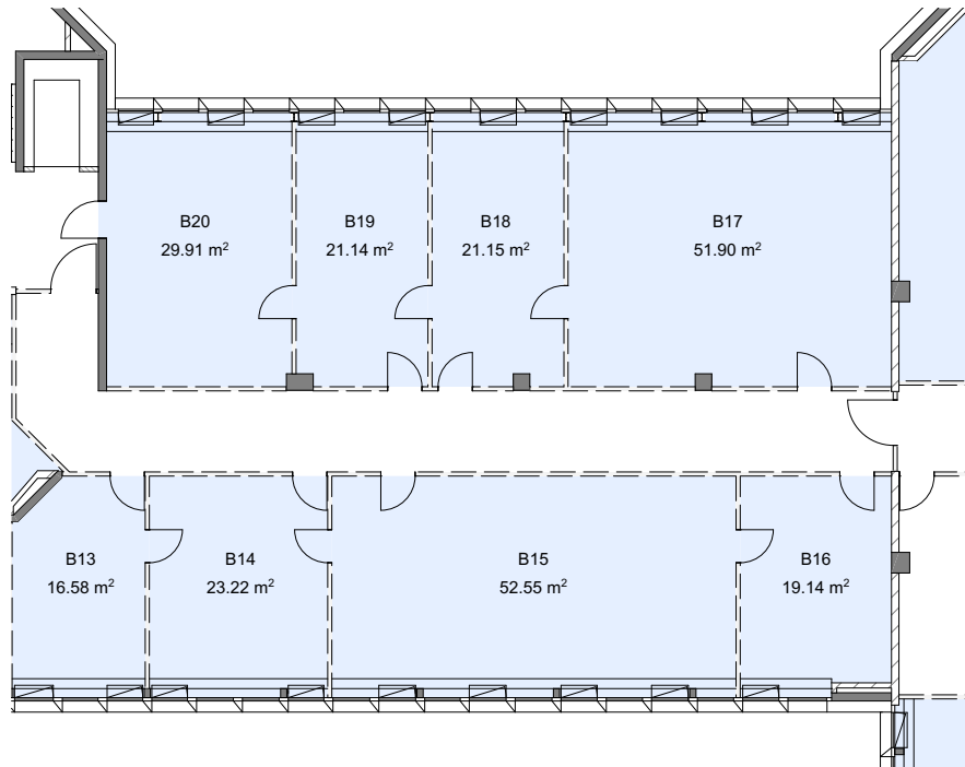
GRUNDRISS ETAGE 2
